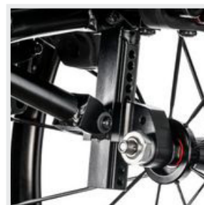
Vario element.
